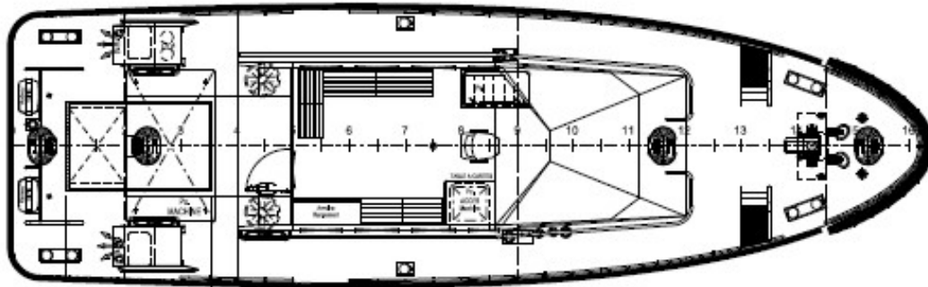
VUE EN PLAN SOUS PONT
