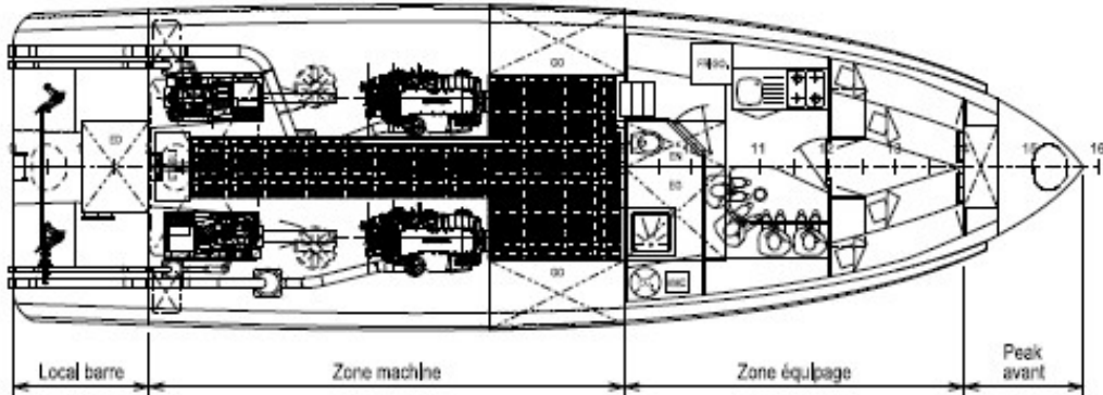
VUE EN PLAN SOUS PONT
